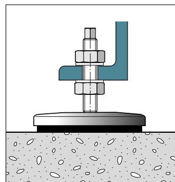
Monteringsexempel Sunnex CM
