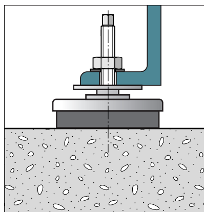
Monteringsexempel Sunnex OSM
