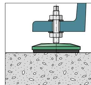
Monteringsexempel Sunnex SM
